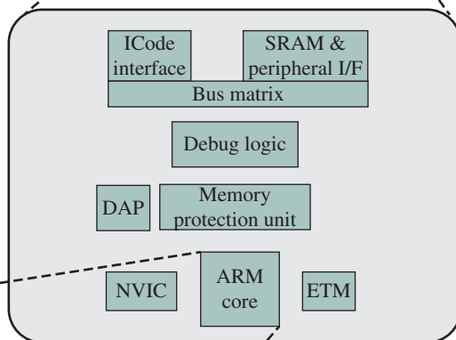
Cortex-M3 Processor
